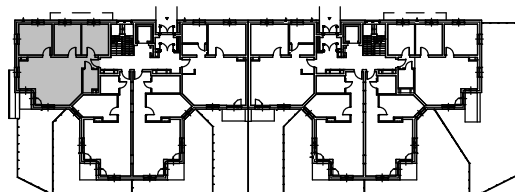
SCHEMAT BUDYNKU
